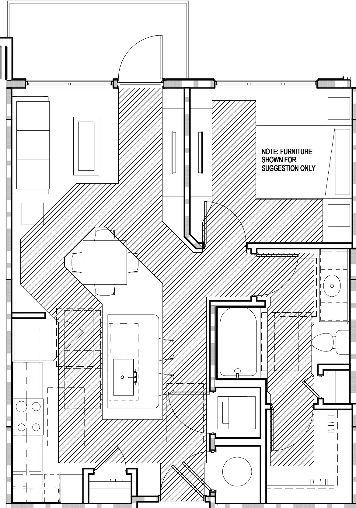
4 UNIT A1 FHA PLAN SCALE: 1/4" = 1'-0"
