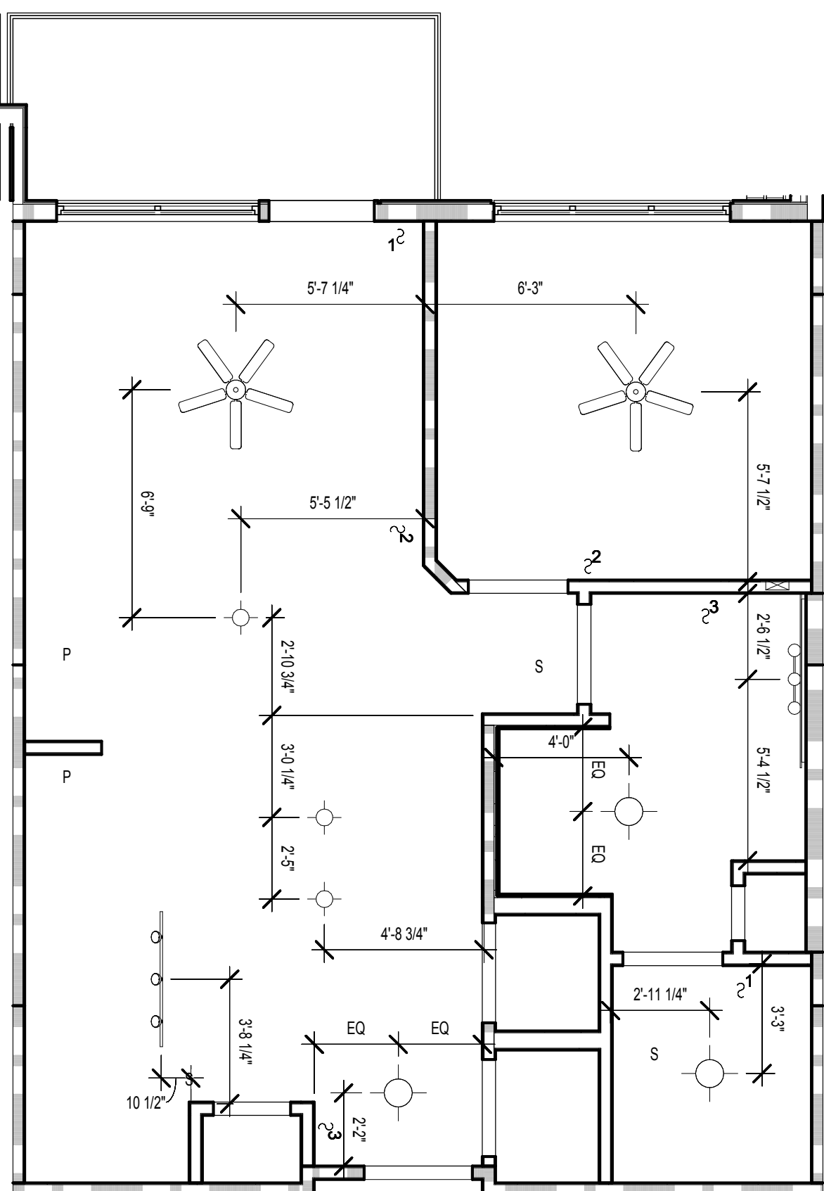
2 UNIT A1 RCP SCALE: 1/4" = 1'-0"
