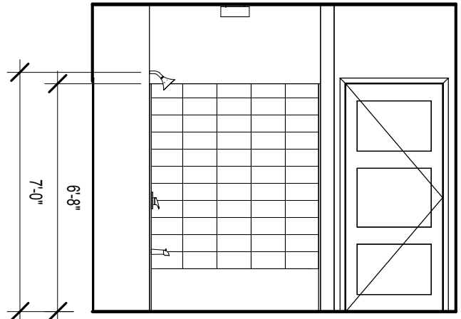
10 UNIT A1 - BATHROOM TUB ELEVATION SCALE: 1/4" = 1'-0"
