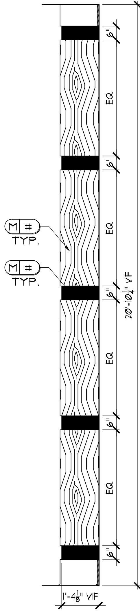
A1.1 ID.601 SECTION SCALE: 1/2" = 1'-0"
