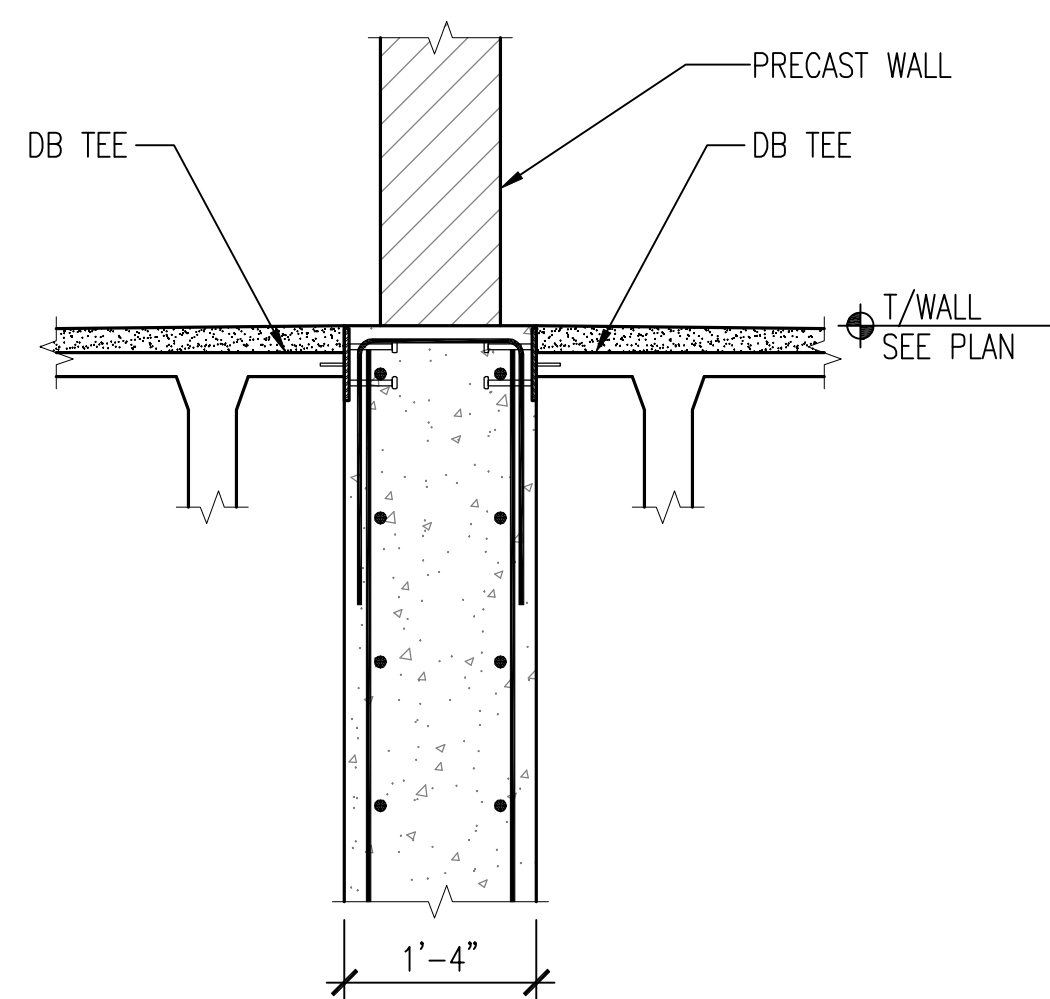
17 SECTION SCALE: 3/4" = 1'-0"
