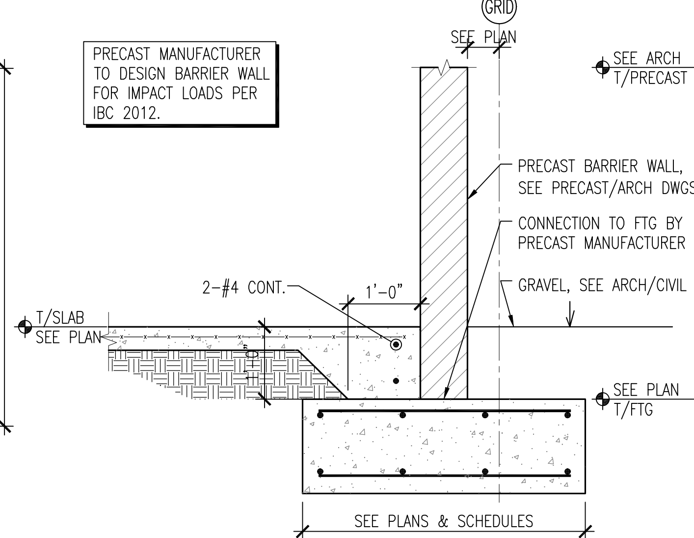
1 SECTION @ EDGE OF SLAB SCALE: 3/4" = 1'-0"
